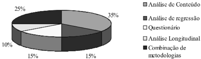
Figura 3: Metodologia utilizada
